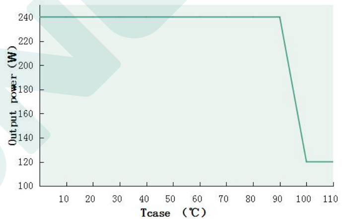
Output power VS Tcase (DL-240W-A/P/X-MXG)
