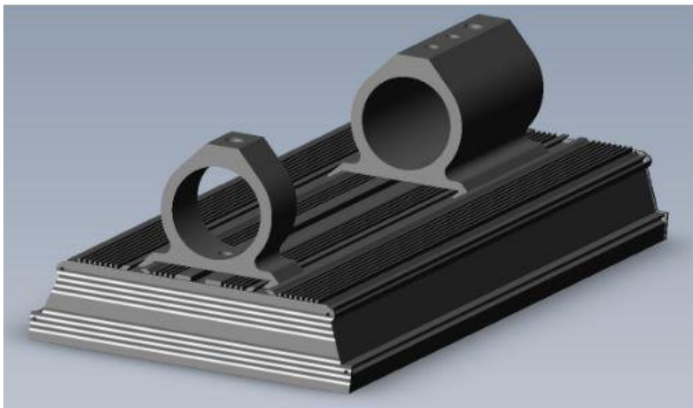
Корпус светильника из профиля ТПК-006 в сборе
