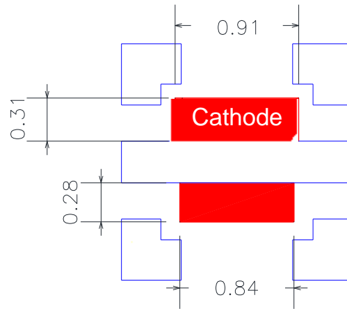
< Bottom >
