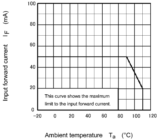
Fig. 11.1 I_F - T_a
