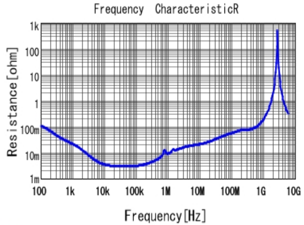
■ KRM55WR71E686MH01 R DCOV, 25degC
