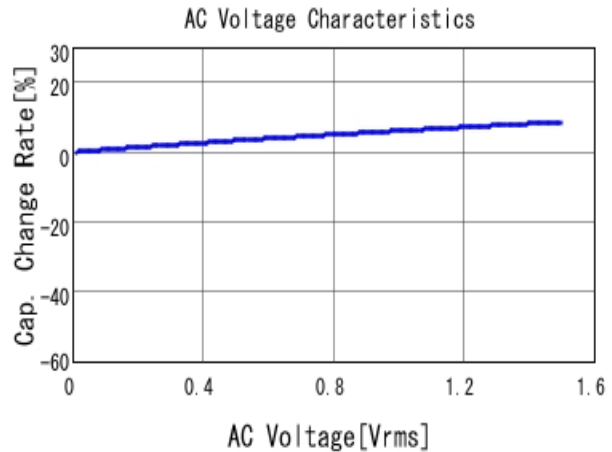
■ KRM55WR71E686MH01 C-AC Voltage capchange, DCOV, 25.0d
