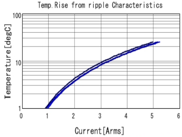
KRM55WR71E686MH01 Temp. rise ■ 50kHz ■ 100kHz ■ 300kHz
