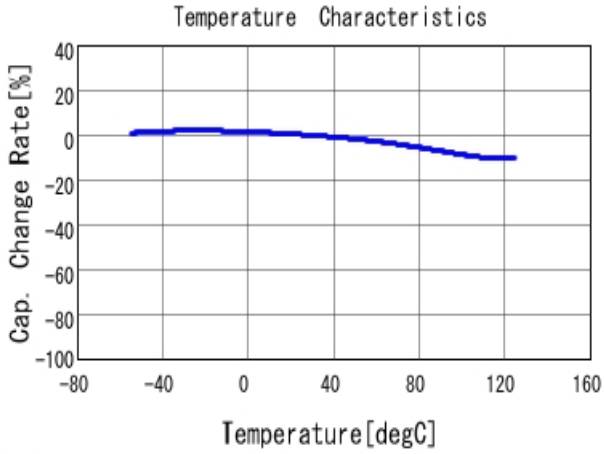
■ KRM55WR71E686MH01 C-Temp. capchange, DCOV, ACO, 5Vrms
