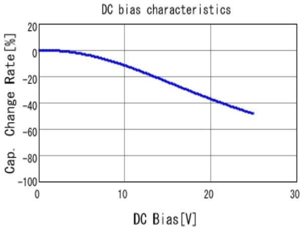
■ KRM55WR71E686MH01 C-DC bias capchange, 25.0degC, AC0.
