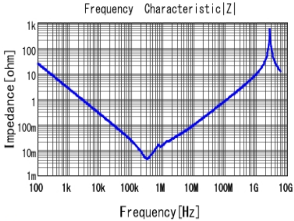
■ KRM55WR71E686MH01 |Z| DCOV, 25degC
