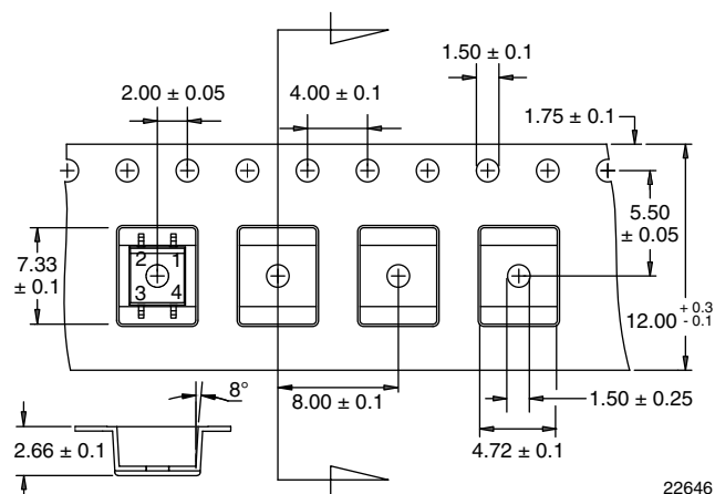
Fig. 13 - Tape Dimensions
