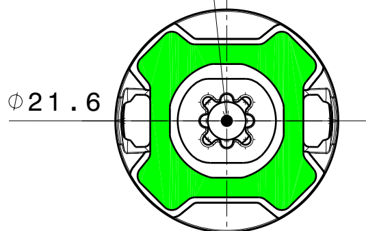
Bottom view Scale: 2:1
