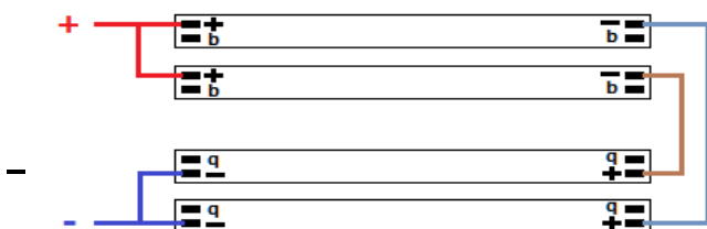
Включение 4-х модулей без разъема по схеме:
