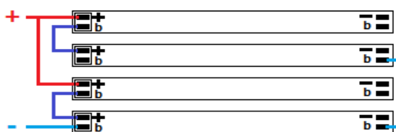
Включение 4-х модулей с разъемом DL250 по схеме:
