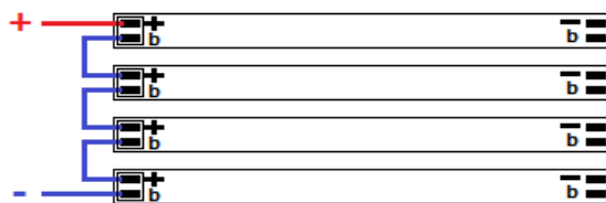
Последовательное включение 4-х модулей с разъемом DL250
