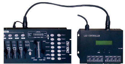
Рис. 4. Подключение DMX-консоли для управления контроллером.
