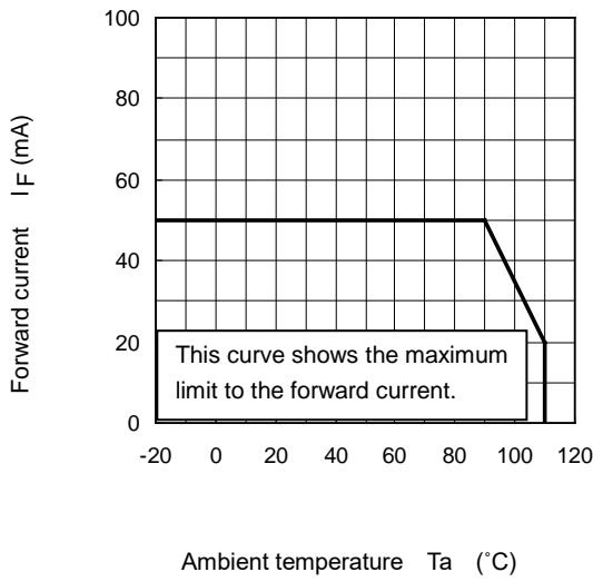
I_F - T_a
