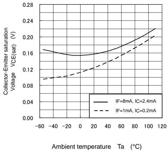
V_{CE(sat)} - T_a
