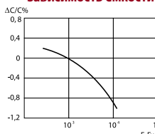
Частотная зависимость емкости
