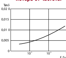
Зависимость тангенса угла потерь от частоты
